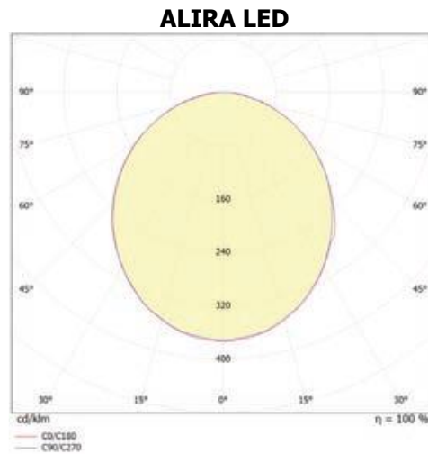
Curba de distribuție a intensității luminoase [Cd/1000lm]
