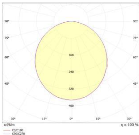
Curba de distribuție a intensității luminoase [Cd/1000lm]
